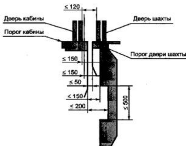
Рисунок 3 - Расстояние между элементами кабины и шахты
